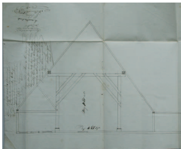
> Bestek met bouwtekening van een Westfriese stulp te Venhuizen 1832 (nominatie 6, Gré Bakker-Bruijn)
